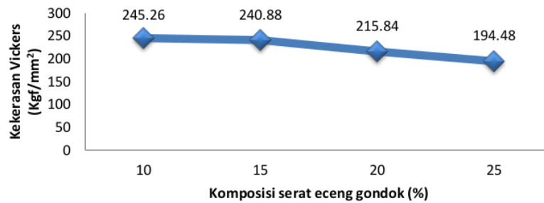
Gambar 4. Data hasil uji kekerasan
