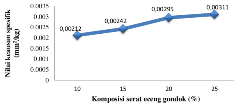
Gambar 5. Data hasil uji keausan
