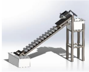
Gambar 1.1 desain prototipe PLTMH
