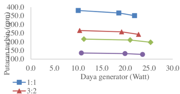
Gambar 1.1 Hubungan Perbandingan diameter puli terhadap putaran turbin dan daya generator
