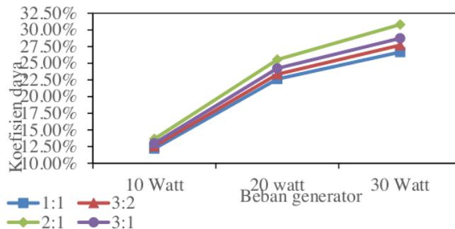
Gambar 1.2 Hubungan Perbandingan diameter puli terhadap efisiensi
