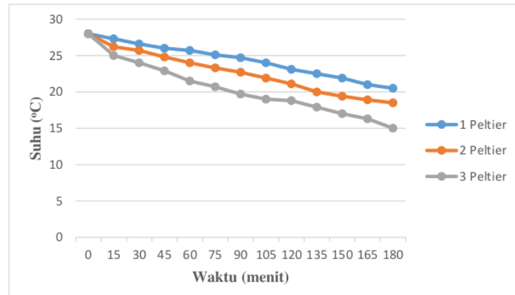
Gambar 8. Grafik Pengujian Masing-Masing Peltier
