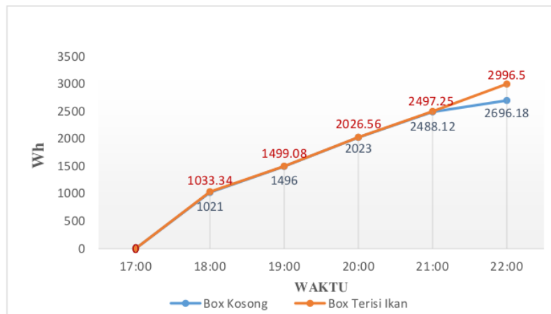
Gambar 14. Gambar Grafik Penggunaan Energi Tanpa Pompa
