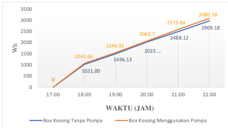
Gambar 16. Grafik Energi Listrik Box Kosong Tanpa Pompa dan Box Kosong Menggunakan Pompa
