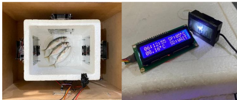
Gambar 11. Pengujian Menggunakan Ikan Tanpa Pompa
