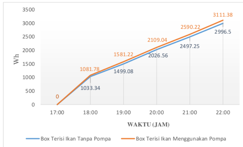
Gambar 17. Grafik Energi Listrik Box Terisi Ikan Tanpa Pompa dan Menggunakan Pompa
