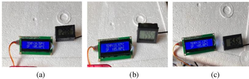
Gambar 9. (a) pengujian 1 peltier, Gambar (b) pengujian 2 peltier, Gambar (c) pengujian 3 peltier
