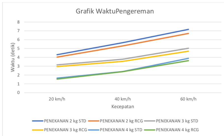
Gambar 1 Grafik Hasil Pengujian Waktu Pengereman
