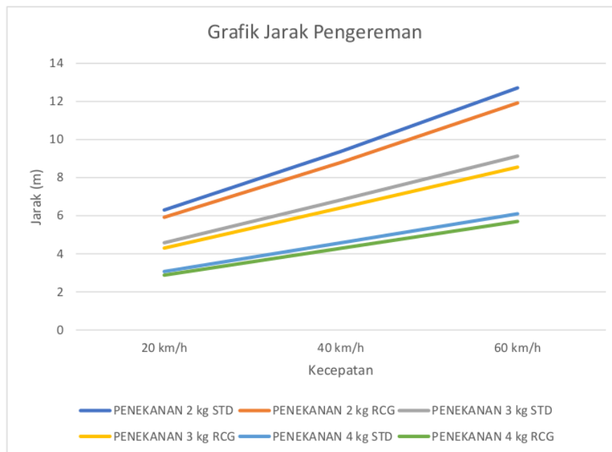
Gambar 2 Grafik Hasil Pengujian Jarak Pengereman
