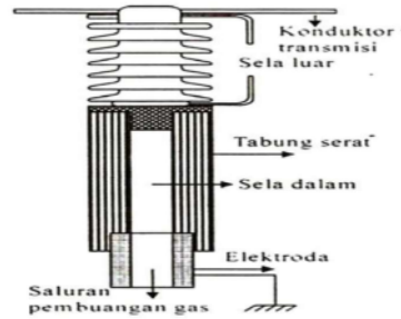
Gambar 1 Elemen arrester jenis eksplusi atau tabung
