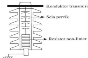
Gambar 2 Elemen Arrester jenis katup
