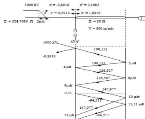
Gambar 5 Diagram tangga kondisi arrester tidak ada dan ada
