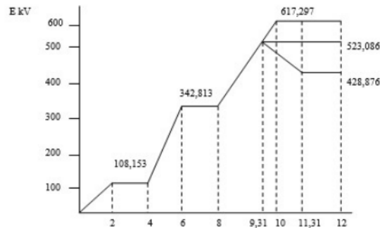
Gambar 6 Tegangan Kondisi Arrester tidak ada dan ada
