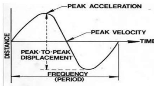
Gambar 1 Karakteristik Getaran
