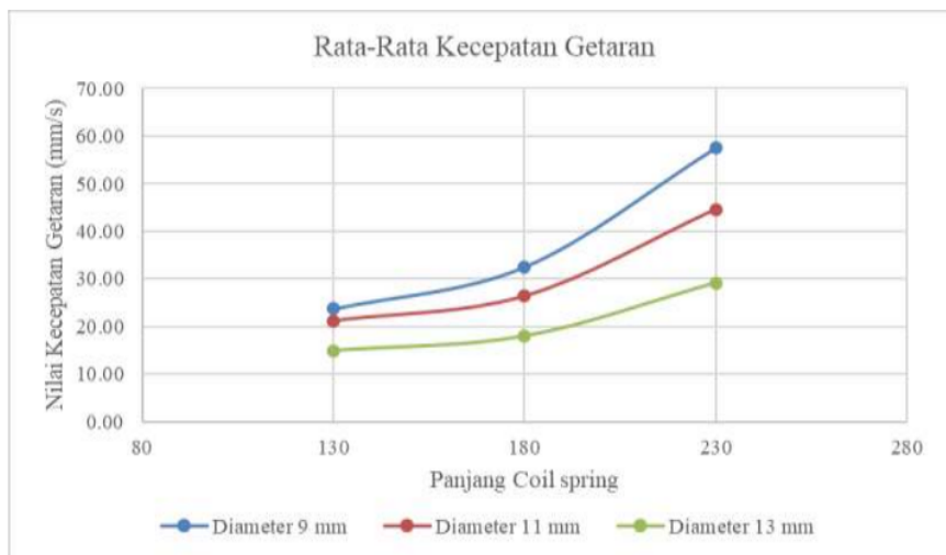
Gambar 4 Grafik Pengujian
