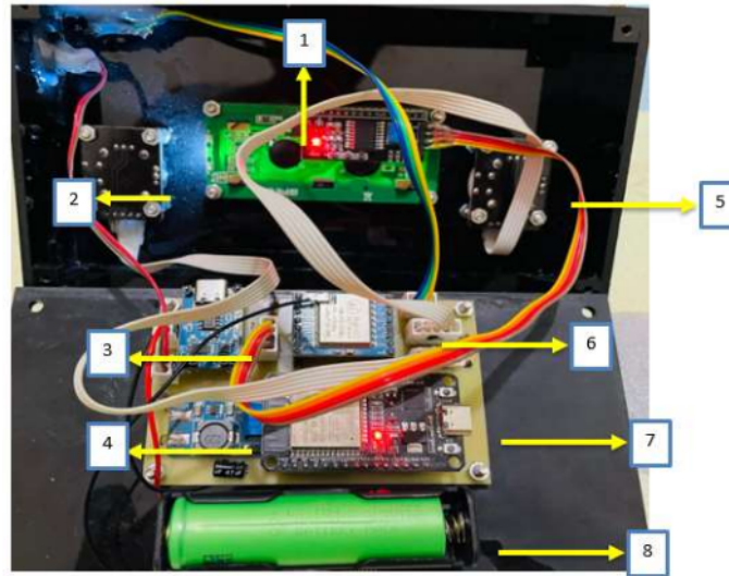
Gambar 4. 7 Perakitan komponen joystick
