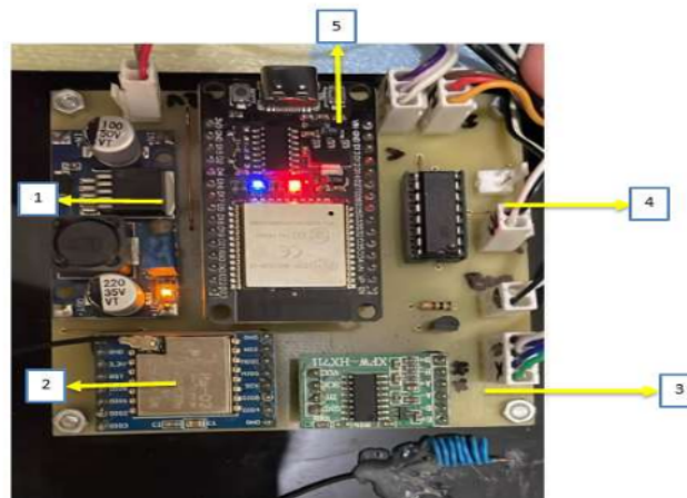
Gambar 4. 8 Perakitan komponen pada crane
