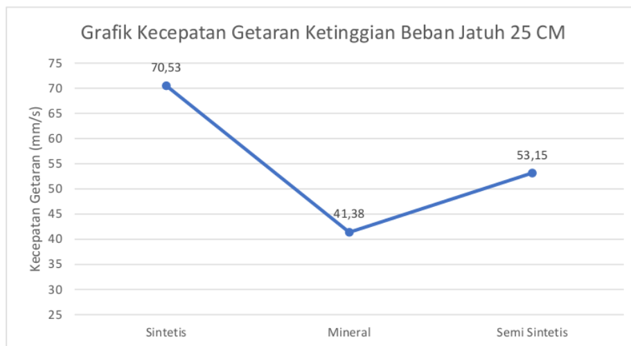
Gambar 4.3 Grafik Kecepatan Getaran Ketinggian Beban Jatuh 25 Cm.
