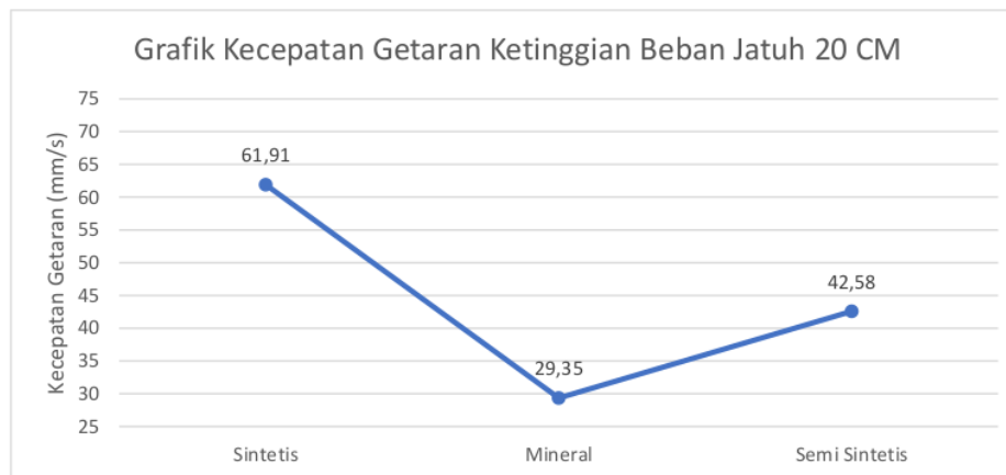
Gambar 4.2 Grafik Kecepatan Getaran Ketinggian Beban Jatuh 20 Cm.
