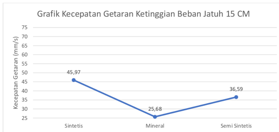
Gambar 4.1 Grafik Kecepatan Getaran Ketinggian Beban Jatuh 15 Cm.
