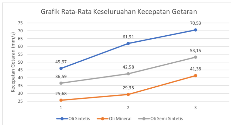
Gambar 4.4 Grafik Rata-Rata Keseluruhan Kecepatan Getaran
