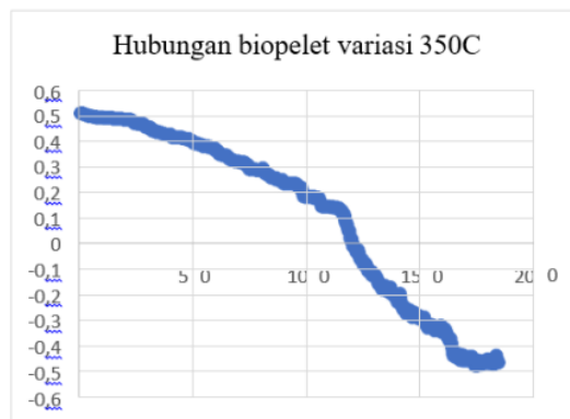
Gambar 8. Uji pembakaran biopellet T350°C
