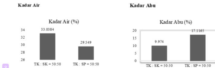
3 Gambar 1. Perbedaan kadar air, abu briket campuran tempurung kelapa, 3 sabut kelapa, dan sekam padi oleh (Vegatama 2022).
