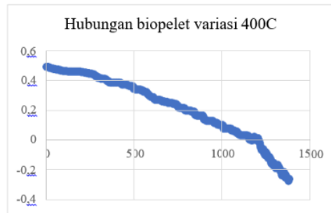
Gambar 7. Uji pembakaran biopellet T400°C
