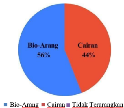
Gambar 5. Distribusi produk T400°C
