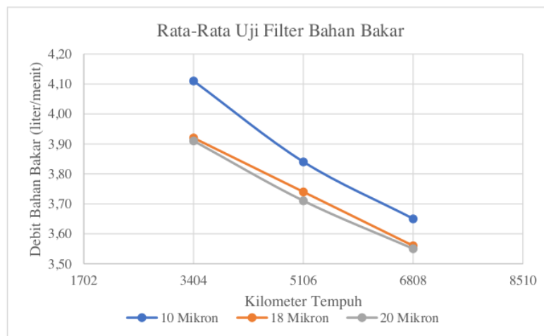
Gambar 4. Rata-Rata Data Uji Filter BB dengan Strainer
