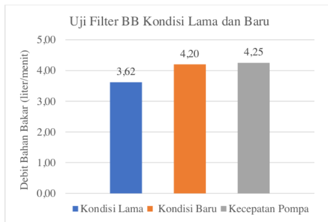
Gambar 2. Uji Filter Lama dan Baru
