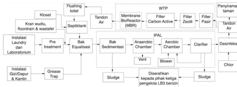
Gambar 4. Diagram Alir Proses Pengolahan Air Limbah
