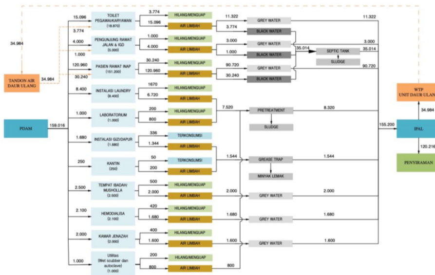
Gambar 3. Diagram Neraca Air Rumah Sakit Umum X
