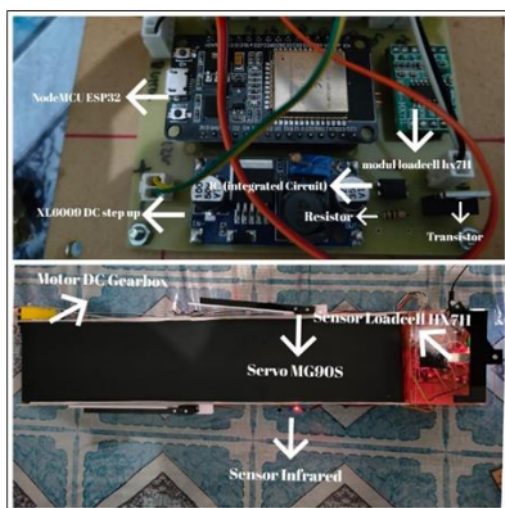
Gambar Hasil keseluruhan perakitan komponen alat pemilah ikan Sumber : Dokumen pribadi
