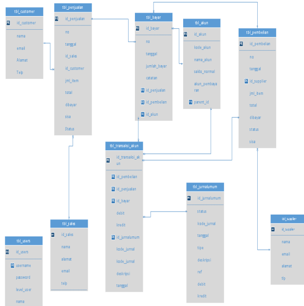
Gambar 6 Gambar Relasi Antar Tabel SIA Web
