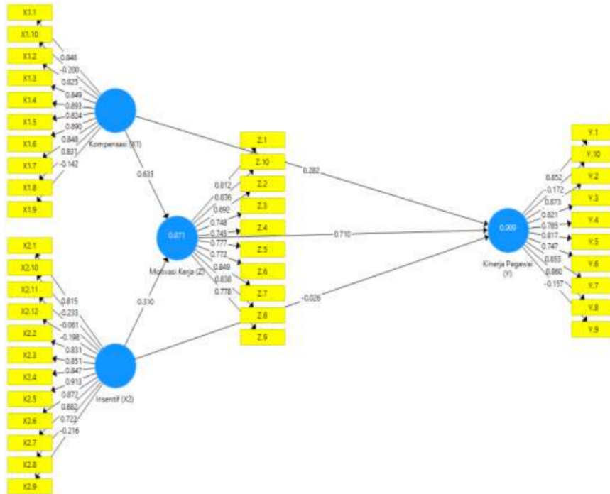
Gambar 2. Hasil Outer Loading Sebelum Eliminasi
