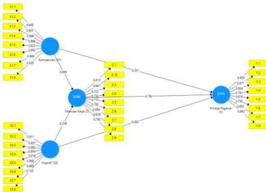
Gambar 3. Hasil Outer Loading Setelah Eliminasi
