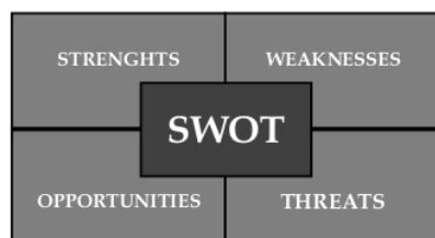
Gambar 2.1 Komponen SWOT
