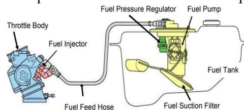
Gambar 1 Komponen Sistem Bahan Bakar EFI
