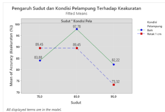
Gambar 5. Grafik Interaksi Antar Variabel Bebas
