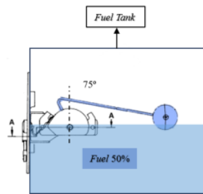
Gambar 8. Skematik Fuel Level Sensor Sudut 75°
