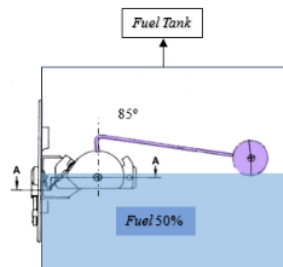
Gambar 7. Skematik Fuel Level Sensor Sudut 85°
