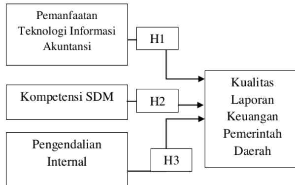
Gambar 2. Kerangka Konseptual
