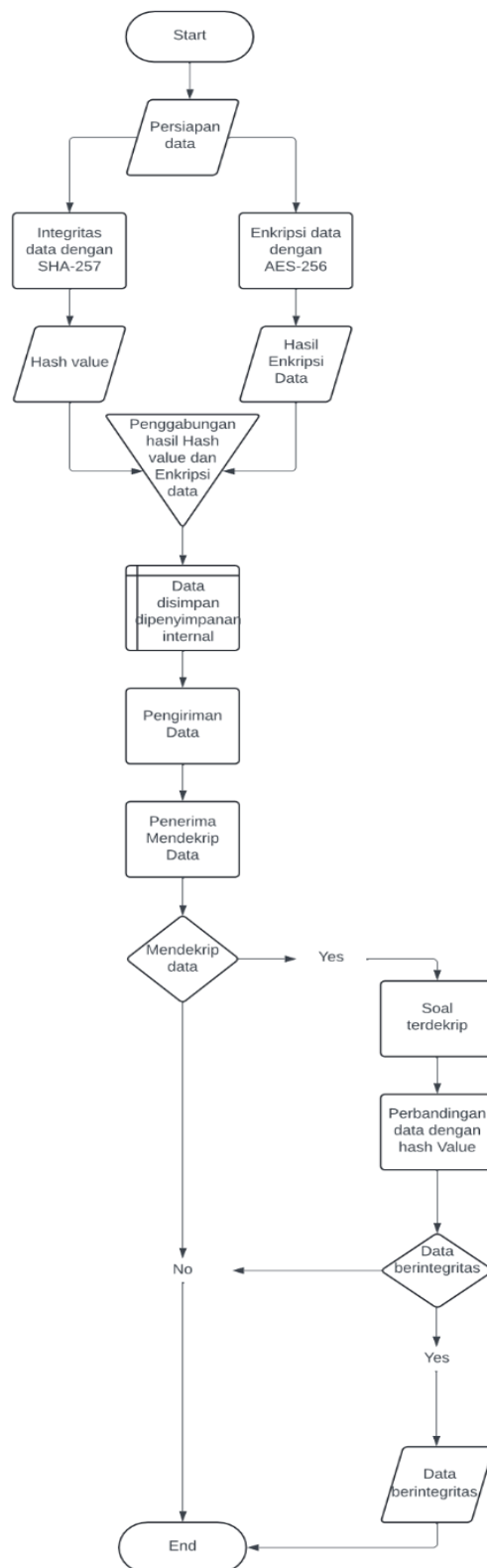
Gambar 24. Flowchart Alur implementasi
