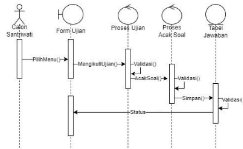
Gambar 4 Sequence Diagram “Mengikuti Ujian CBT dengan Pengacakan Soal Algoritma Fisher Yates ”
