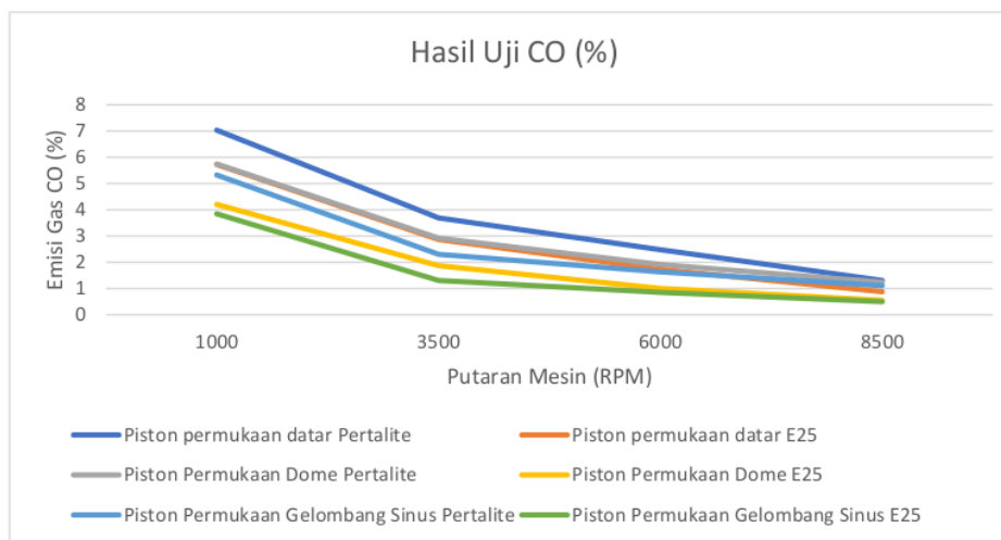
Gambar 3. Grafik Emisi CO
