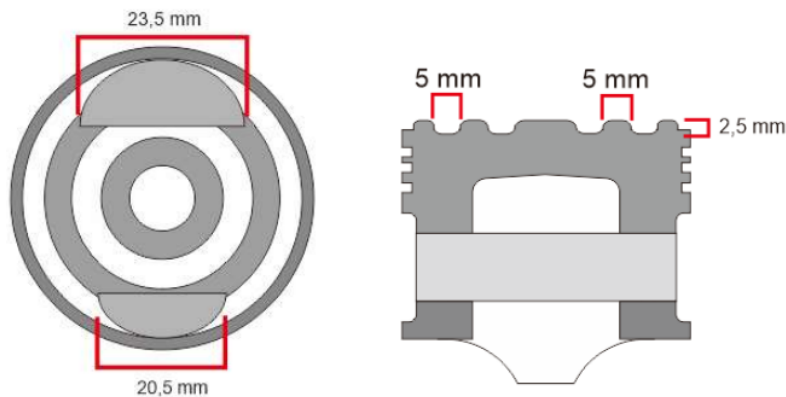
Gambar 2. Ukuran modifikasi piston
