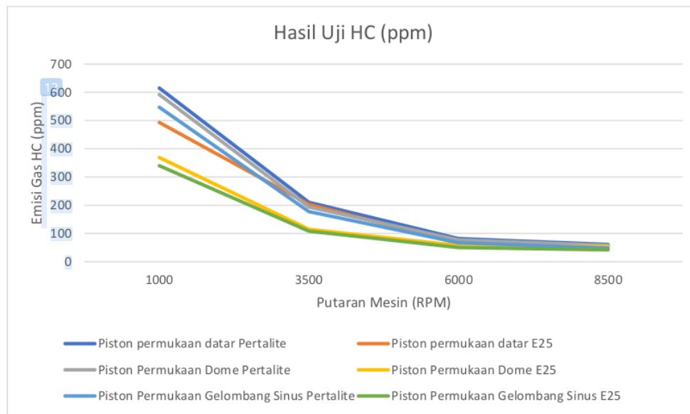
Gambar 4. Grafik Emisi HC
