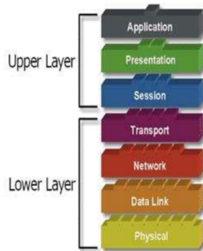
Gambar 1. OSI Layer
