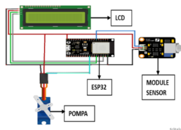
41 Gambar 3.3 Perancangan Alat
