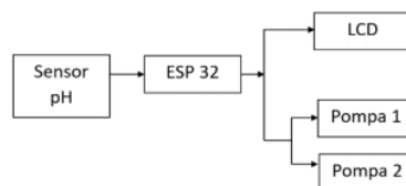
Gambar 3.1 Perancangan Sistem
