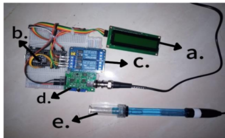
Gambar 4.1Tampilan Keseluruhan Alat
